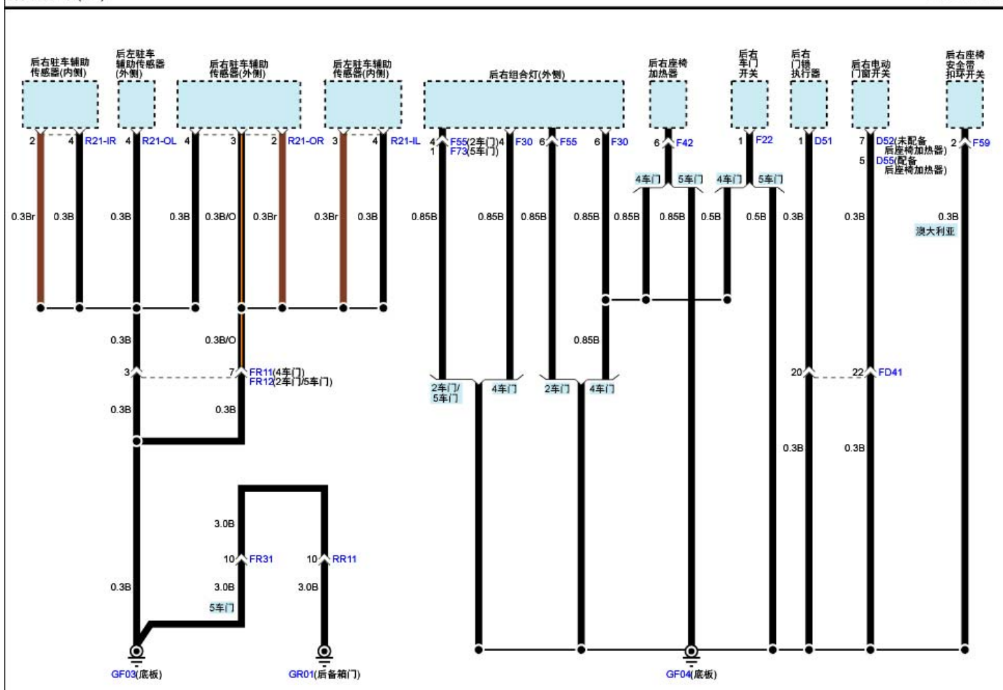
搭铁分布(10)
